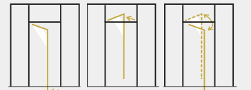
1 vantaux : ouverture intérieure, extérieure et va-et-vient avec parties fixes et imposte
