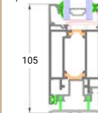
Seuil plat
