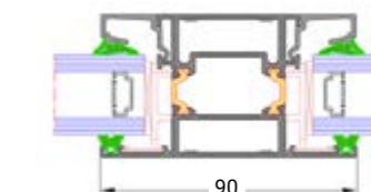
Traverse intermédiaire
