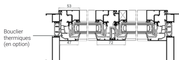
Porte-fenêtre serrure
