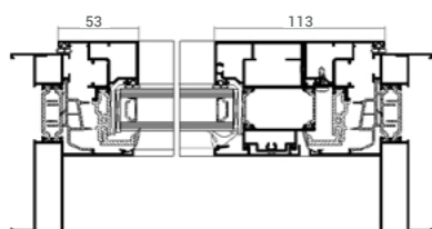
Porte-fenêtre serrure
