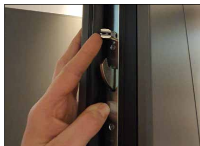
Serrure automatique 5 points à crochets, plus résistante qu'une serrure à rouleaux
