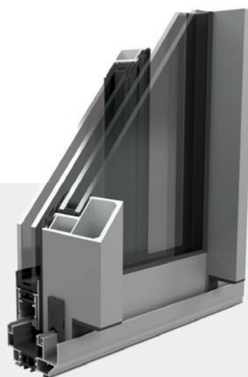
Porte 2 vantaux
