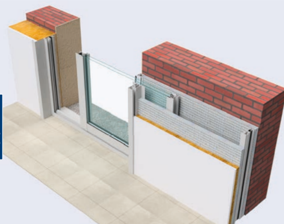
Version isolée
